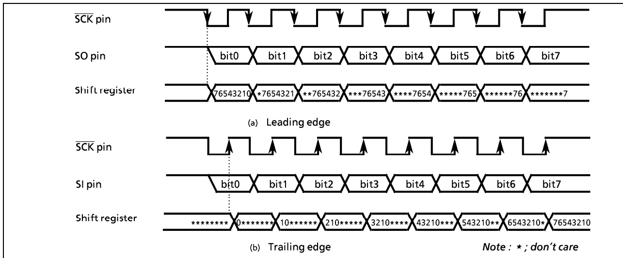
Figure 2-53. Shift Edge
